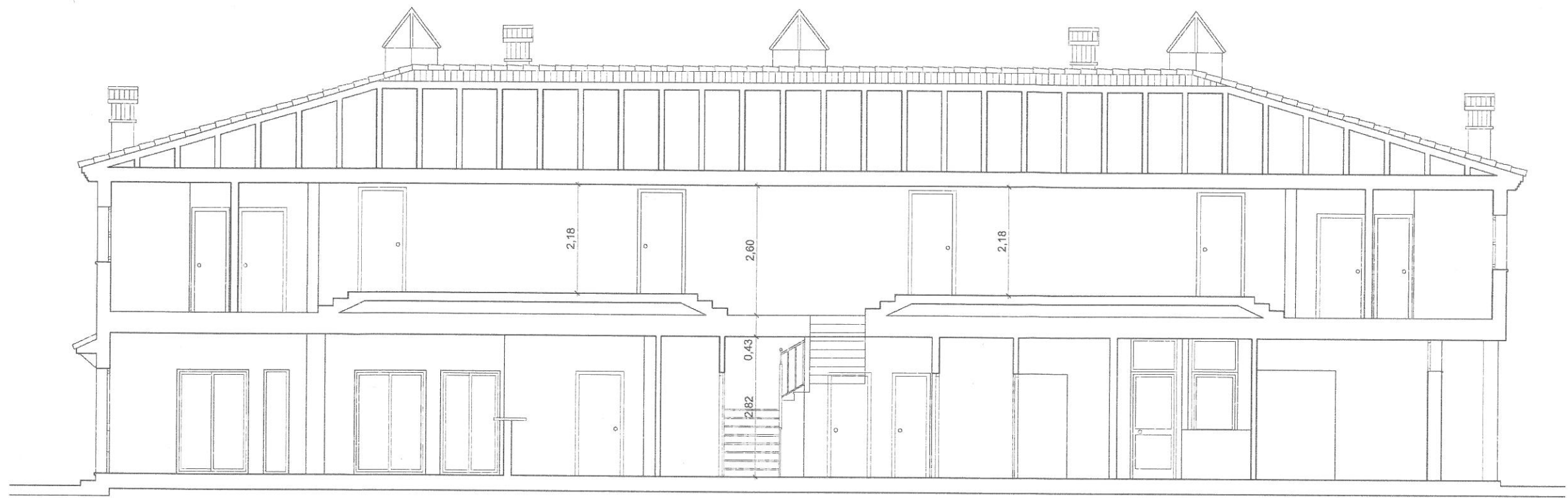
SECCIÓN A-A
