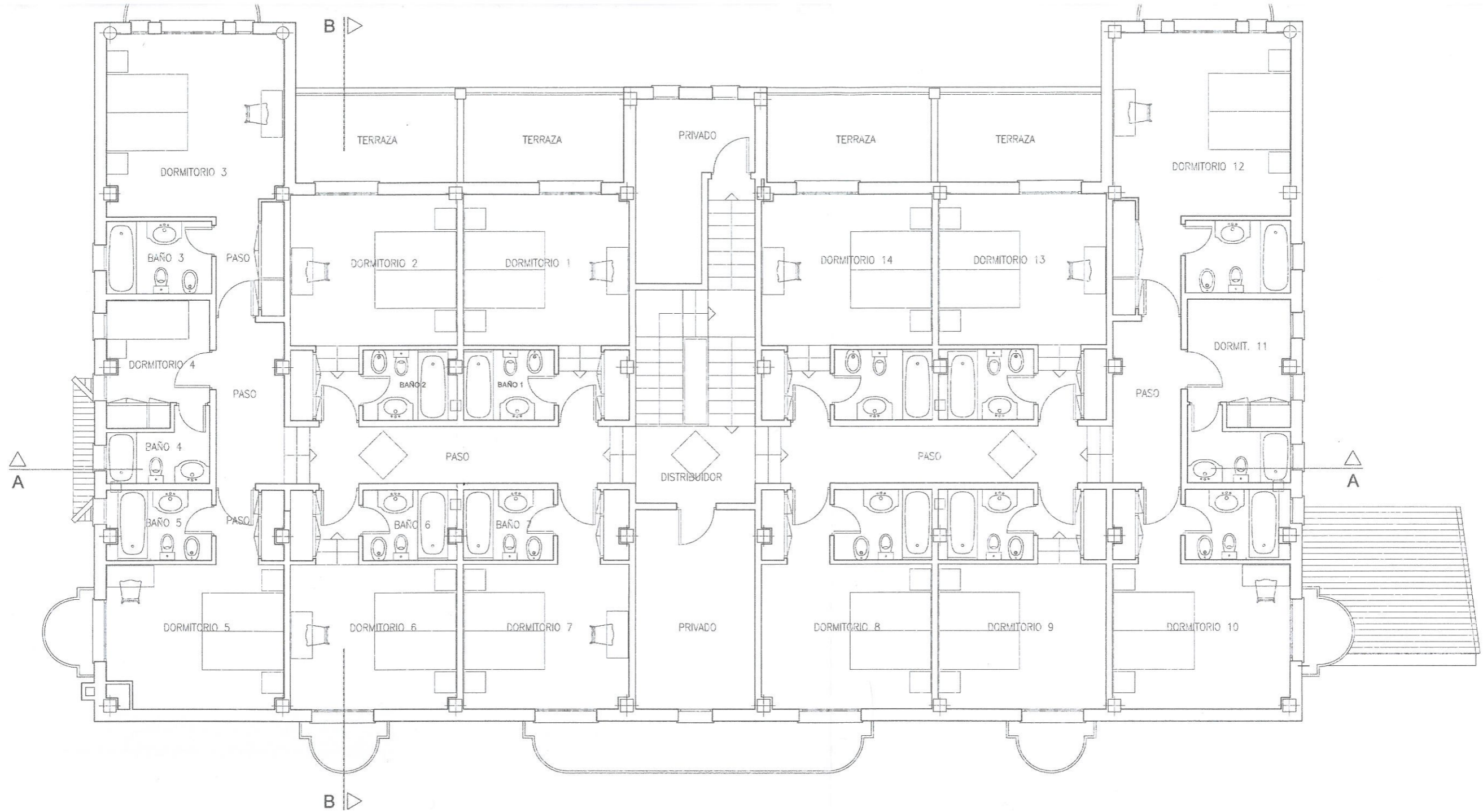
PLANTA ALTA
