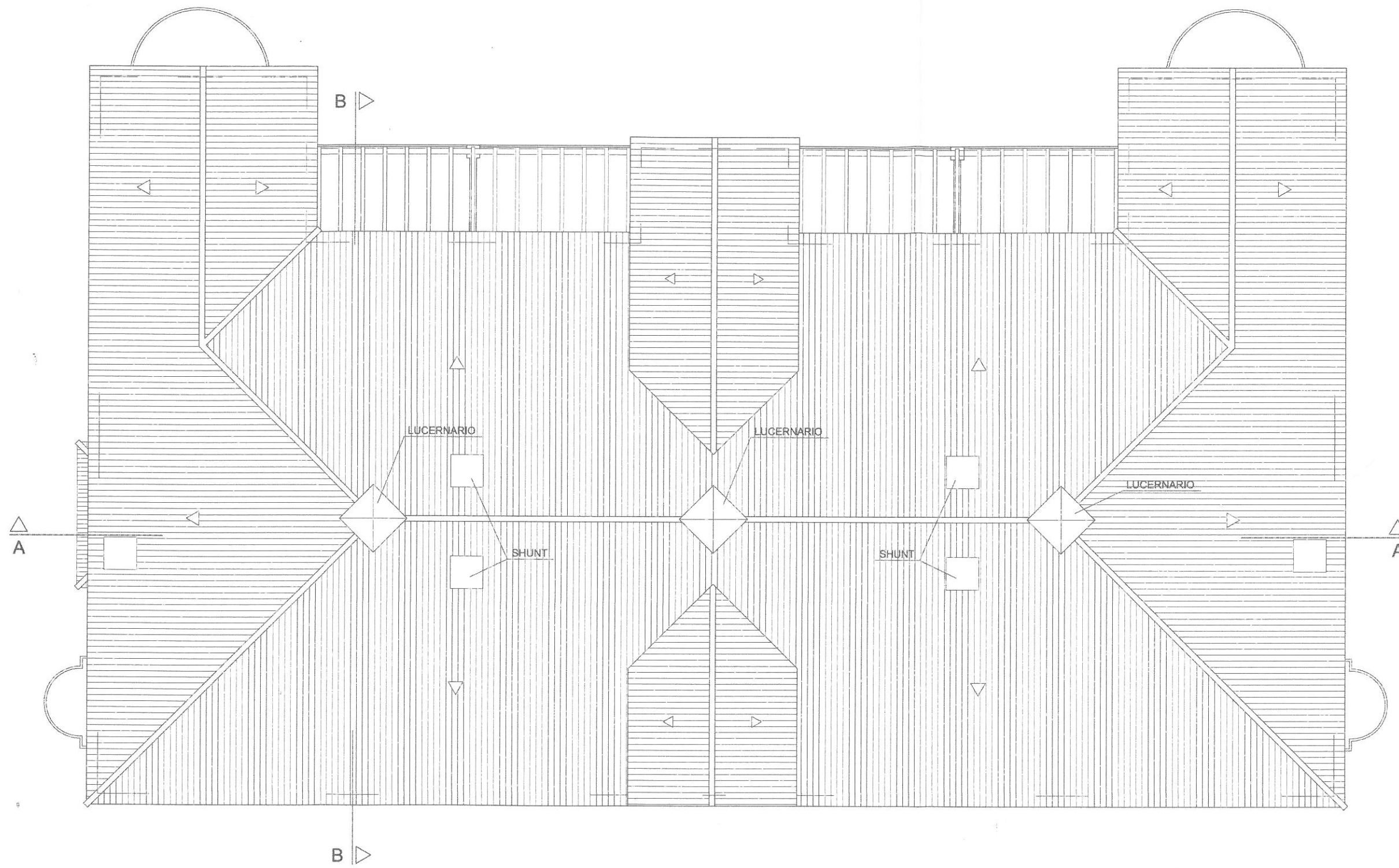
PLANTA ALTA
