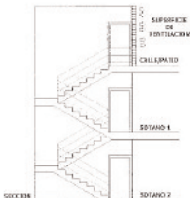
Ventilación de escalera acumulada en Planta Superior con abertura permanente. Superficie mínima 2l = 10A \text{ m}^2 .
