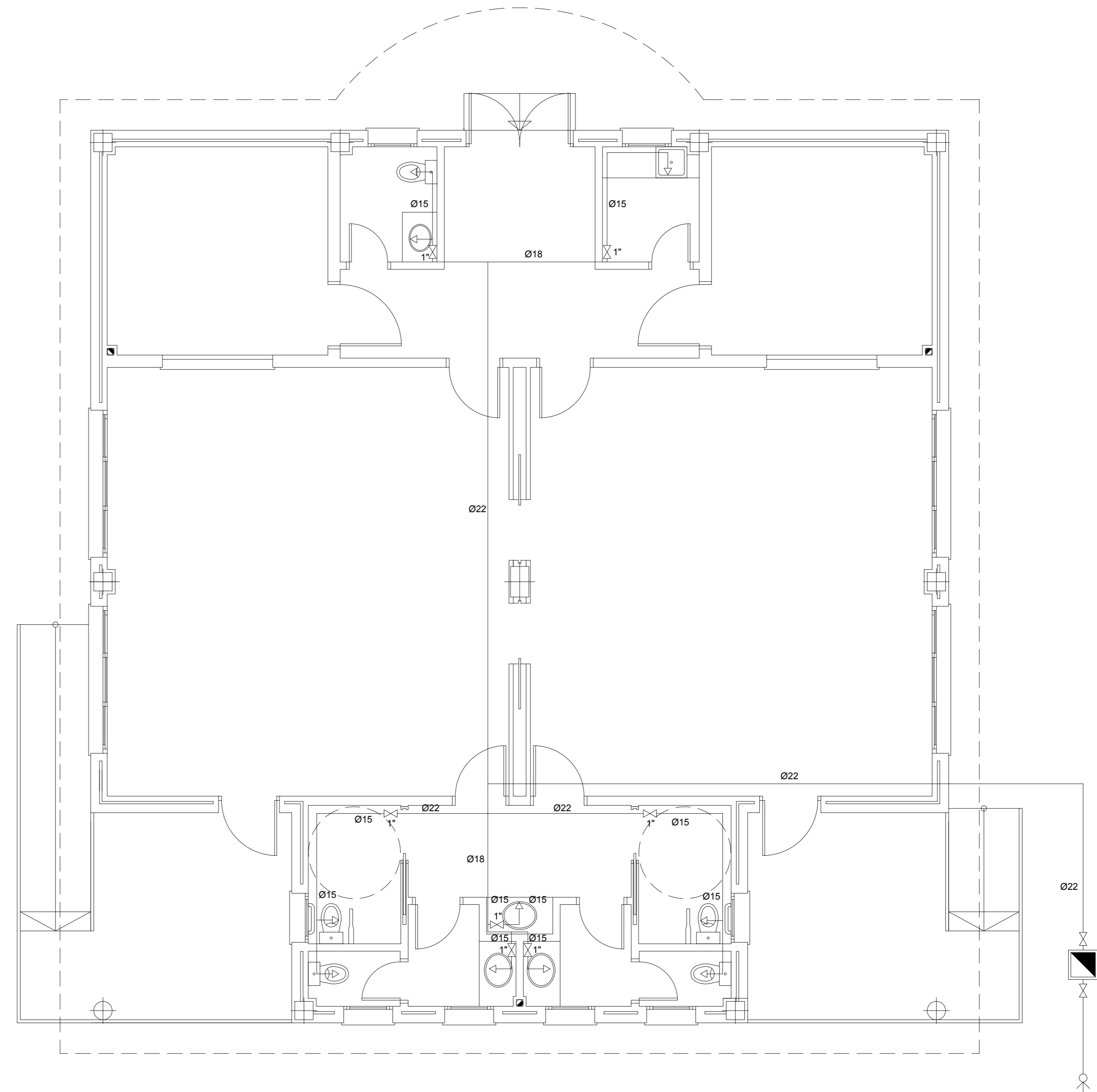
PLANTA BAJA: FONTANERIA
