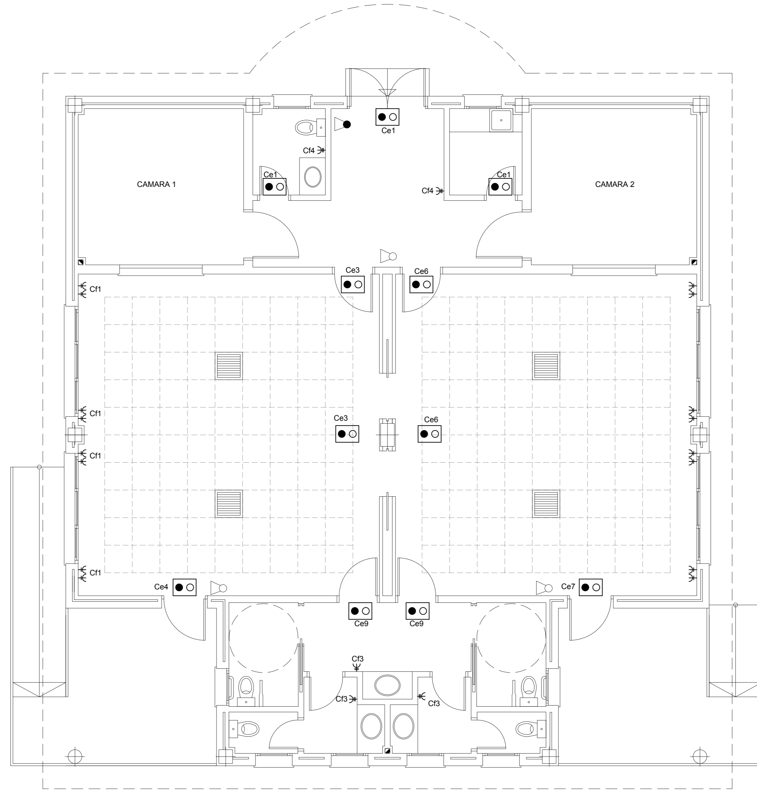
PLANTA BAJA: FUERZA Y CPI
