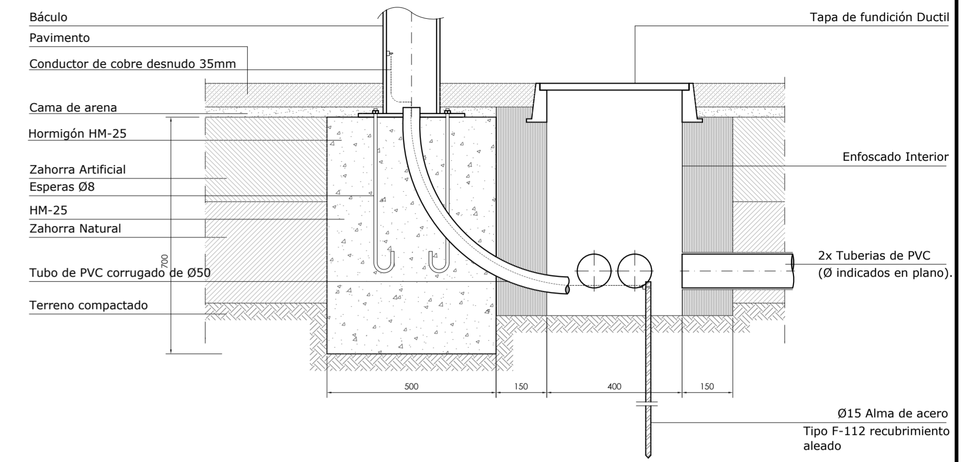
ARQUETA TIPO CON TOMA DE TIERRA Y BASE PARA BÁCULO
