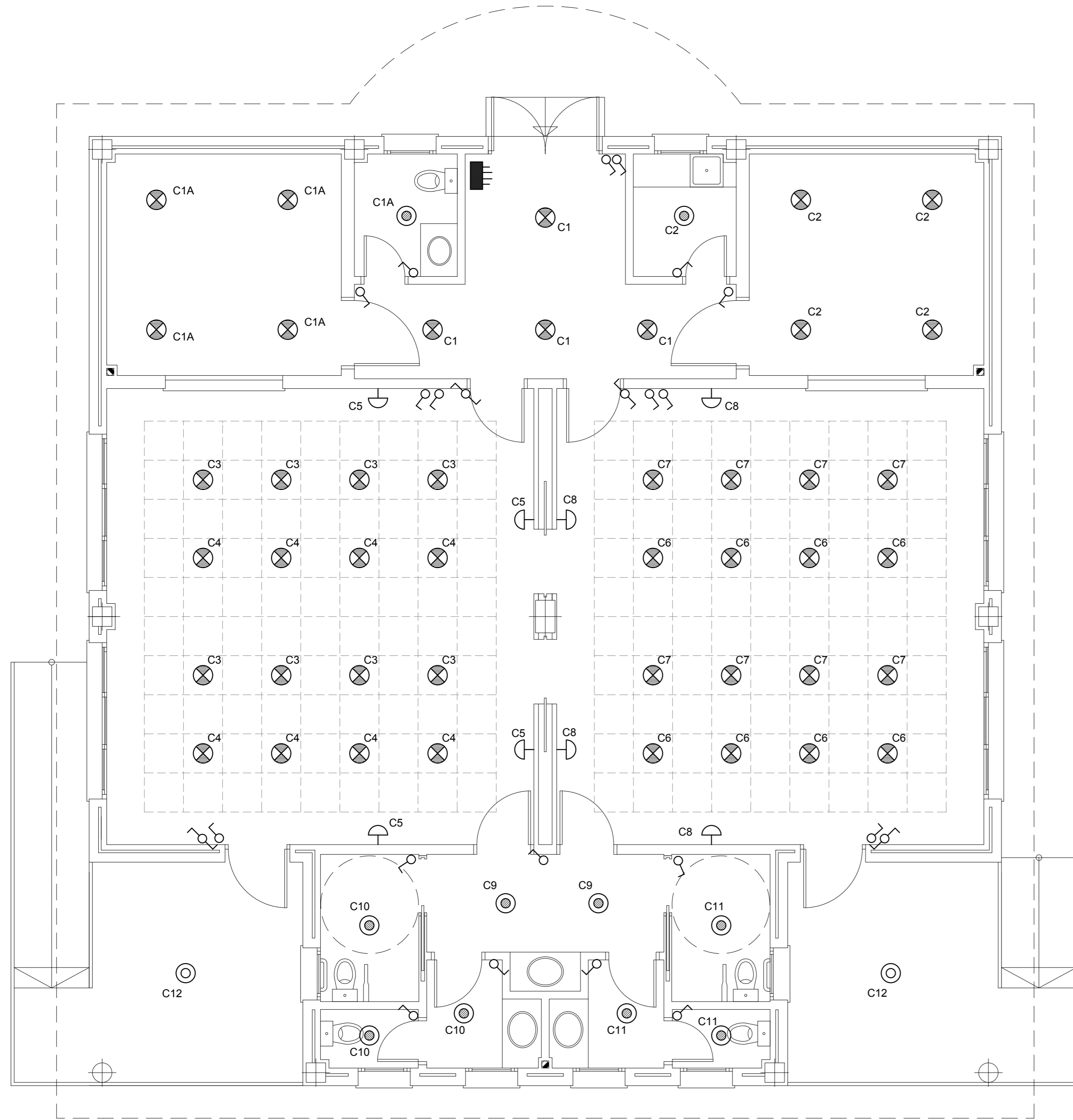
PLANTA BAJA: ALUMBRADO
